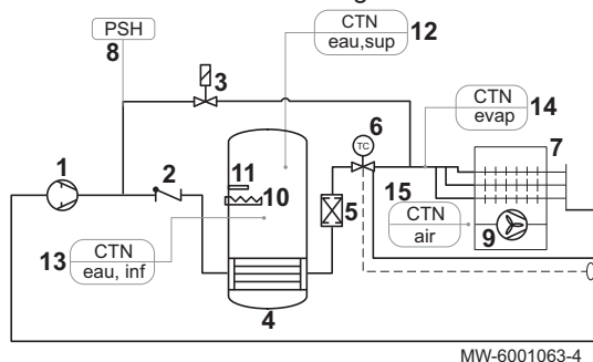
Afb.16 AZORRA Ace 200 - AZORRA Ace 250 met verwarmingselement
