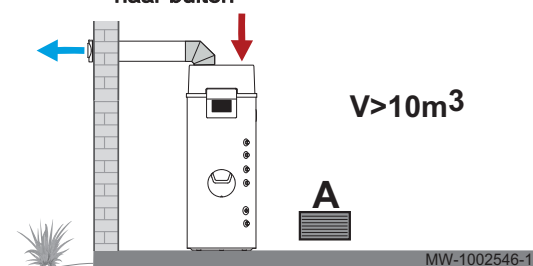
Afb.31 Het toestel zuigt lucht vanuit een gesloten ruimte aan en voert het af naar buiten
