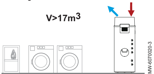
Afb.27 Wasruimte: Het toestel zuigt lucht aan en voert lucht af in een gesloten ruimte.
