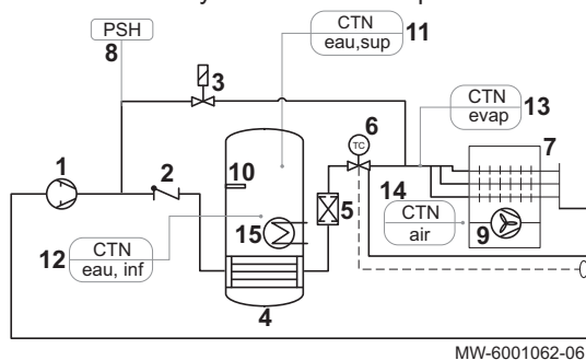
Afb.17 AZORRA Ace 200 H - AZORRA Ace 250 H met verwarmingsspiraal voor hydraulische back-up
