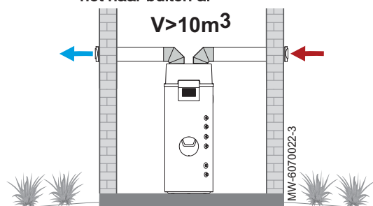
Afb.29 Het toestel zuigt lucht vanuit een gesloten ruimte aan en voert het af naar buiten
