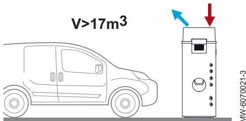
Afb.26 Garage: Het toestel zuigt lucht aan en voert lucht af in een gesloten ruimte
